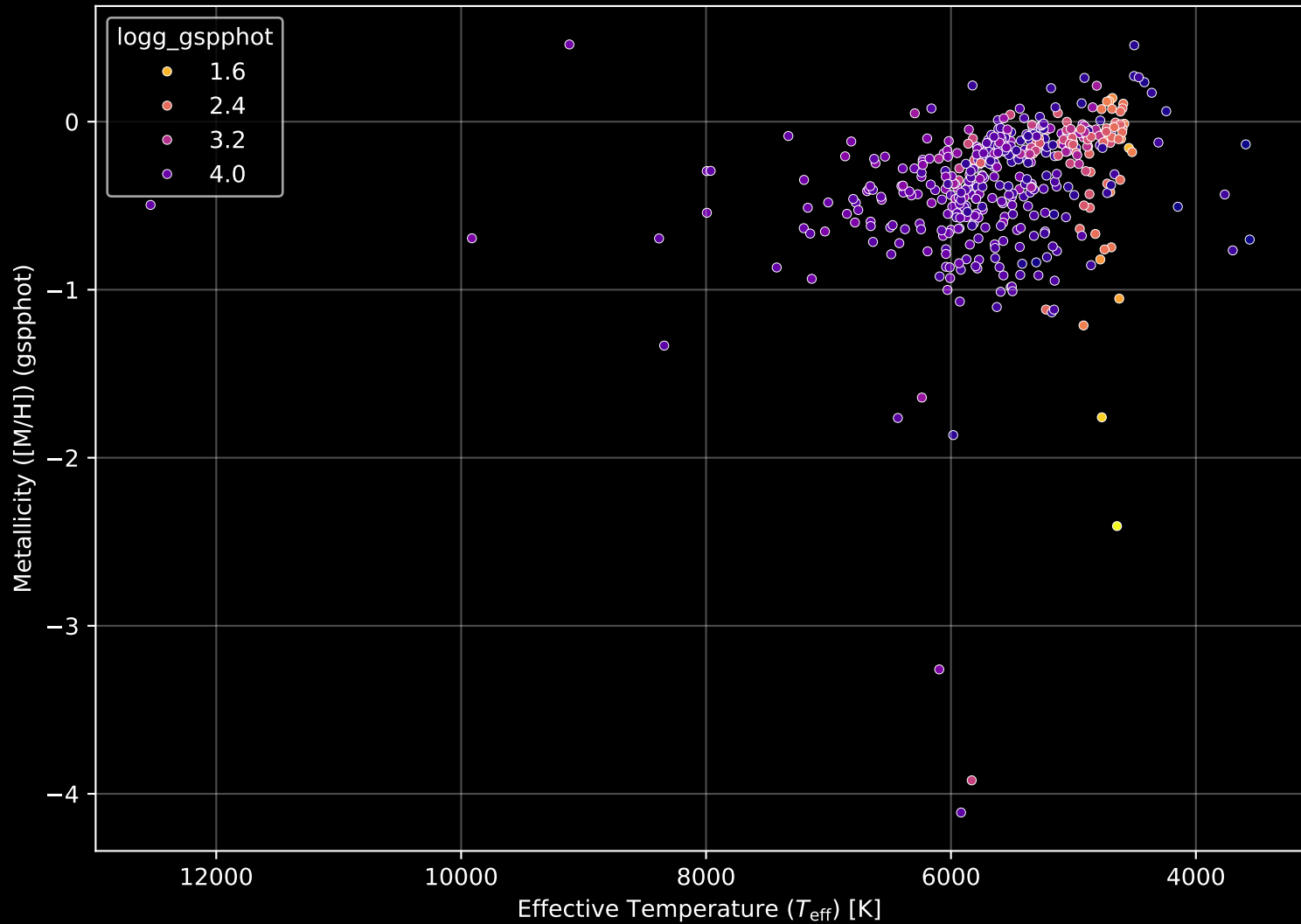
GALAH DR4 Field: [6585] Stellar Population Parameters (n= 457)
