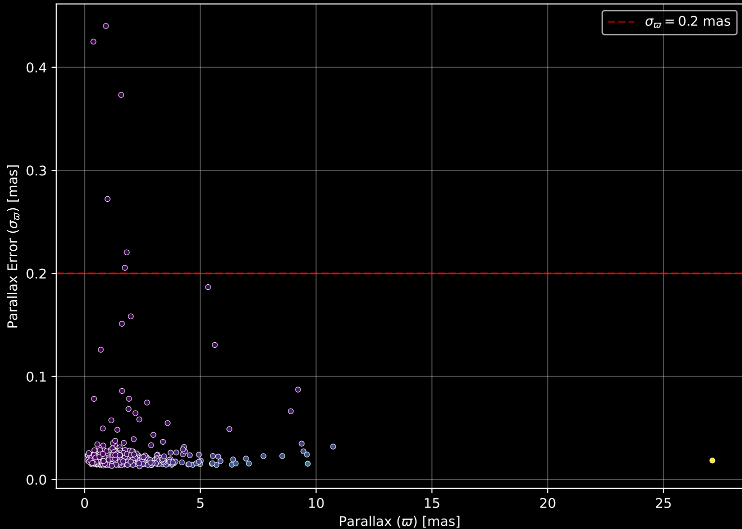
GALAH DR4 Field: [6585] Parallax Quality (n= 457)
