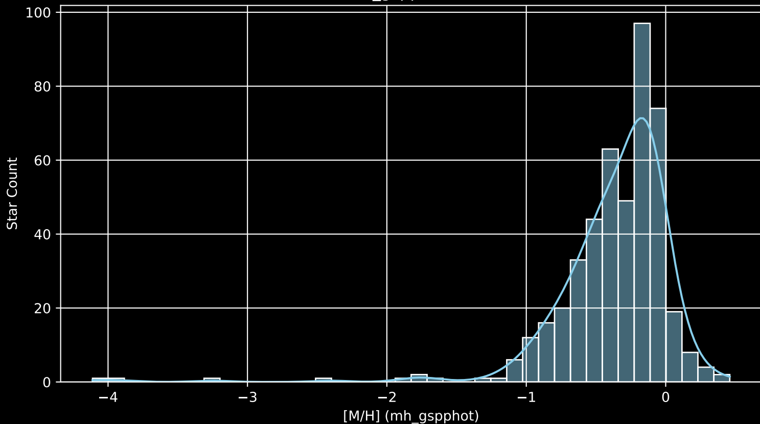
GALAH DR4 Field: [6585] [M/H] (mh_gspphot) (n= 457)
